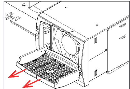
C) Utilice la cubierta como asa para retirar el módulo
