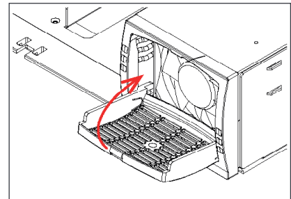
C) Cierre la cubierta encastrando el módulo en su lugar, si resulta difícil, vuelva a realizar el paso B
